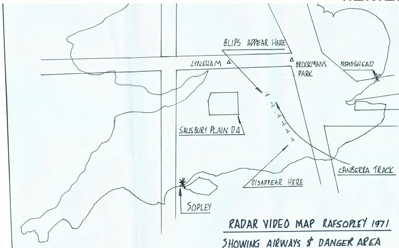
Mapa del área que muestra la pista en el objetivo del radar no identificado. Mapa proporcionado por Alan Turner.
